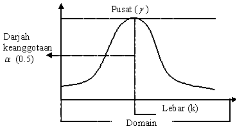
Rajah 3. Ciri Fungsi Lengkuk Gauss
