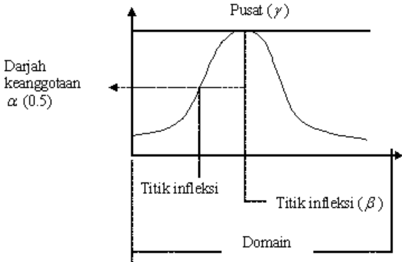
Rajah 2. Ciri Fungsi Lengkung Phi
