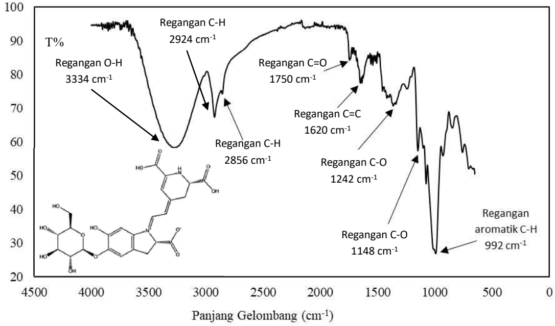
RAJAH 2. Spektrum FTIR ekstrak buah naga
